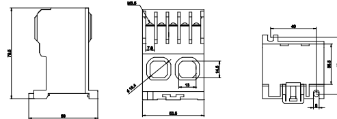
OPR - SS2E / SS2 / UC2 (2홀 관통형) 단위:mm
