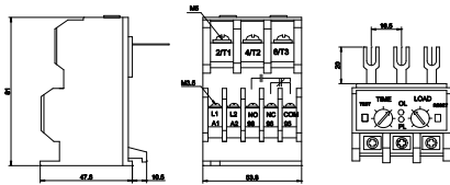
OPR - EP50 (MC 직결형) 단위:mm
