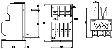
OPR - SP (MC 직결형) 단위:mm
