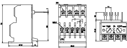
OPR - EP (MC 직결형) 단위:mm
