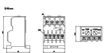
OPR - NPR (전자식 역상 계전기) / GR (전자식 지복계전기) OV (전자식 과전압 계전기) / UV (전자식 부족전압 계전기) 단위:mm
