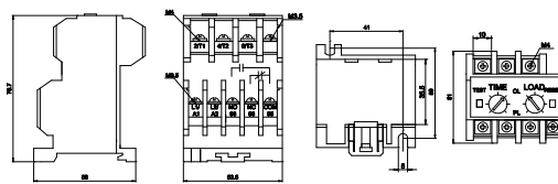
OPR - ES (단자 접속형) / UC (단자접속형) 단위:mm
